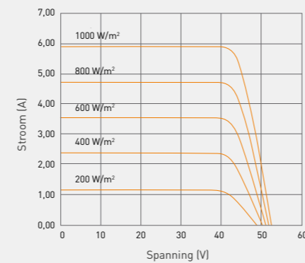
Referentiegegevens voor model VBHN245SJ25 (Celtemperatuur: 25 °C.)
