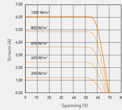
Referentiegegevens voor model VBHN330SJ53 (Celtemperatuur: 25 °C.)
